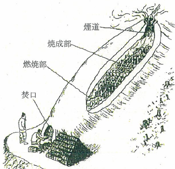
窯の施設の名称と製品を焼くイメージ図 (「図解 技術の考古学」より)
