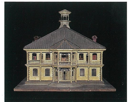
宮城県会議事堂 建築模型 (写真: 東北大学大学院工学研究科都市・建築学専攻提供)
