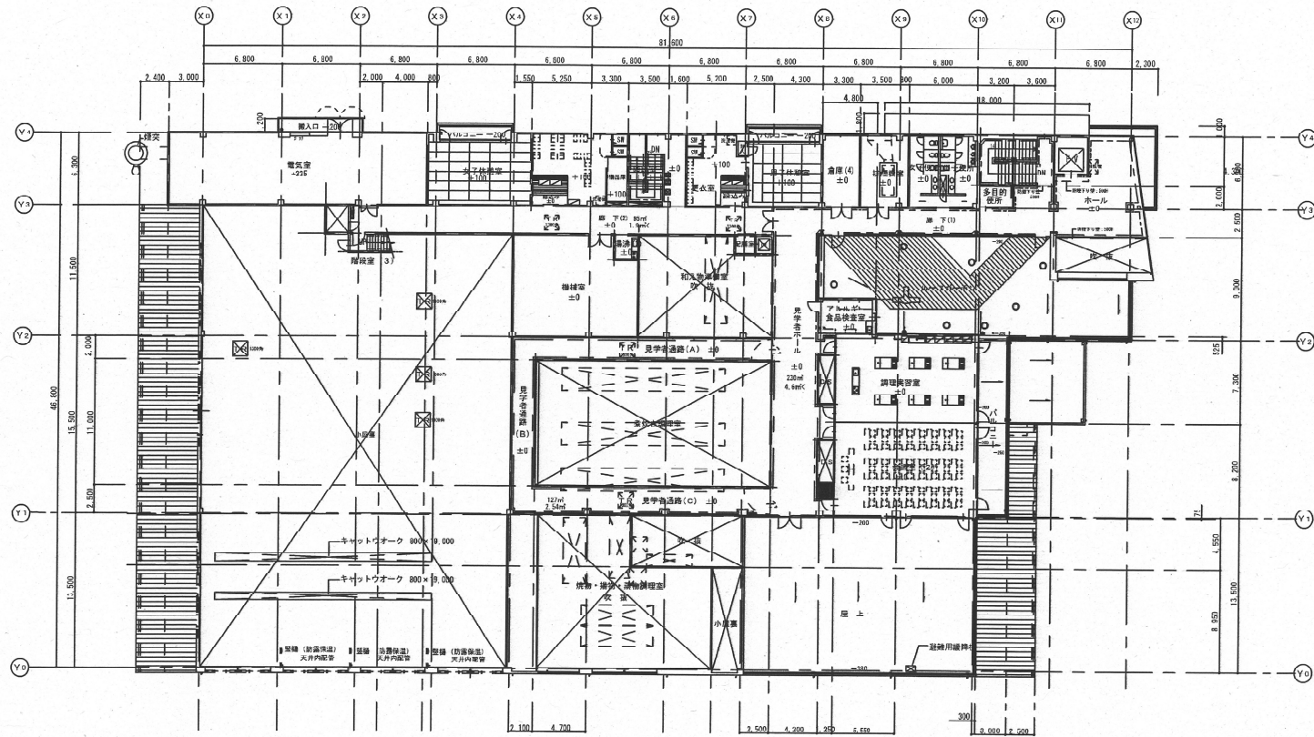
2階 平面図 1:200
