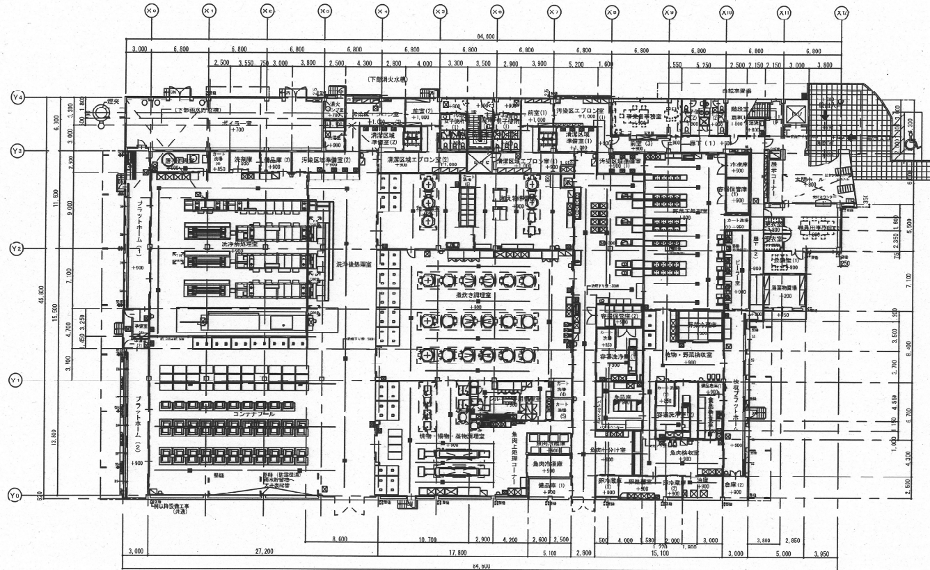
1階 平面図 1:200 ±N: 設計G.L.からの高さを示す --- 千原位置
