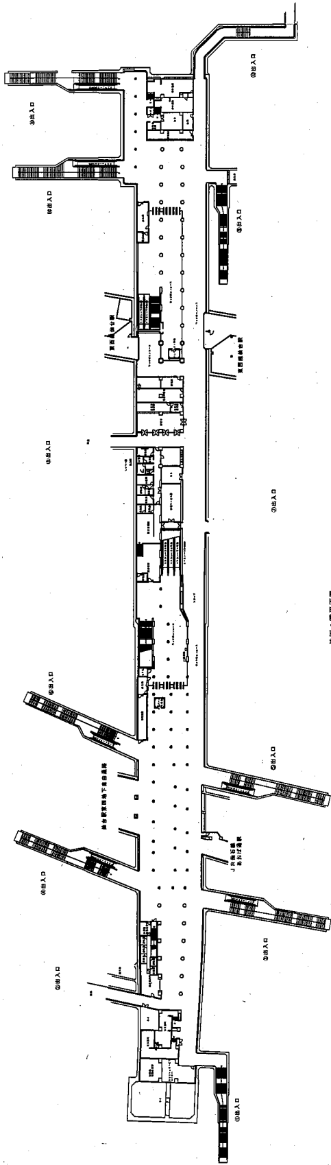
地下1階平面図
