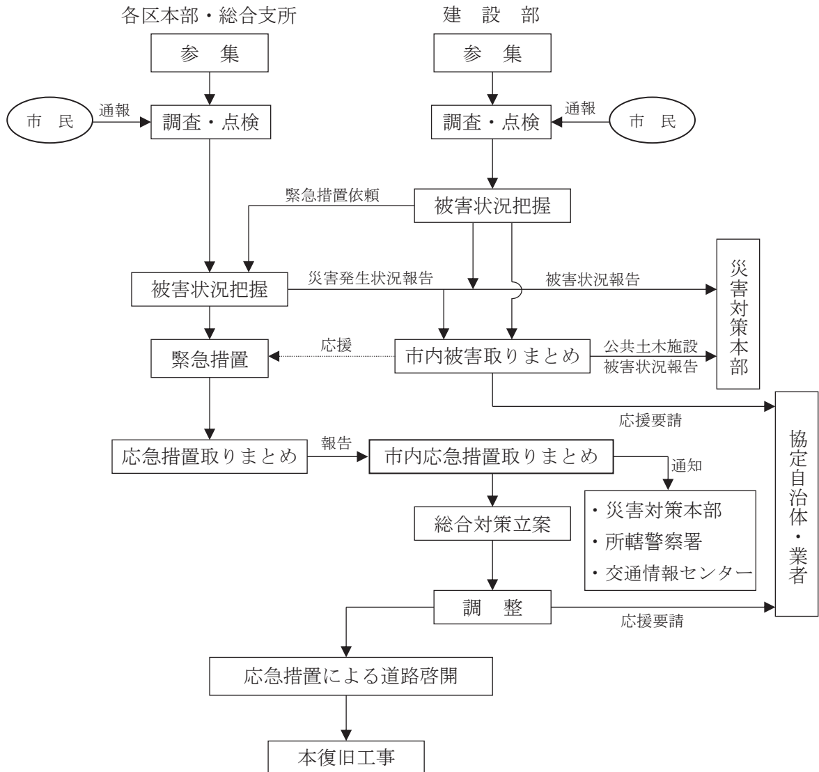
〈道路・橋梁の点検及び応急措置フロー図〉
