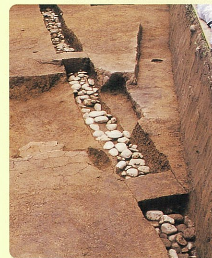
▲写真⑩ 石組の暗渠溝 河原石を組合せて暗渠にしています
